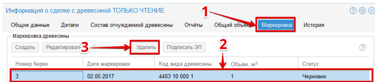
Рисунок 116 – Окно «Информация о сделке с древесиной».
